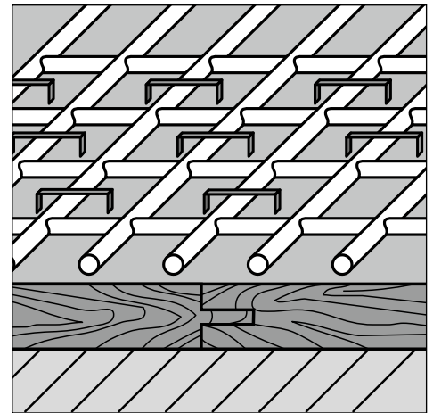
Armierung auf kritischen Untergründen
