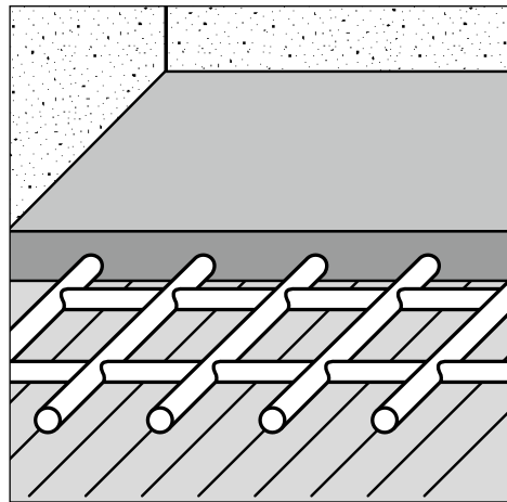
Mörtel- oder Spachtelarmierung
